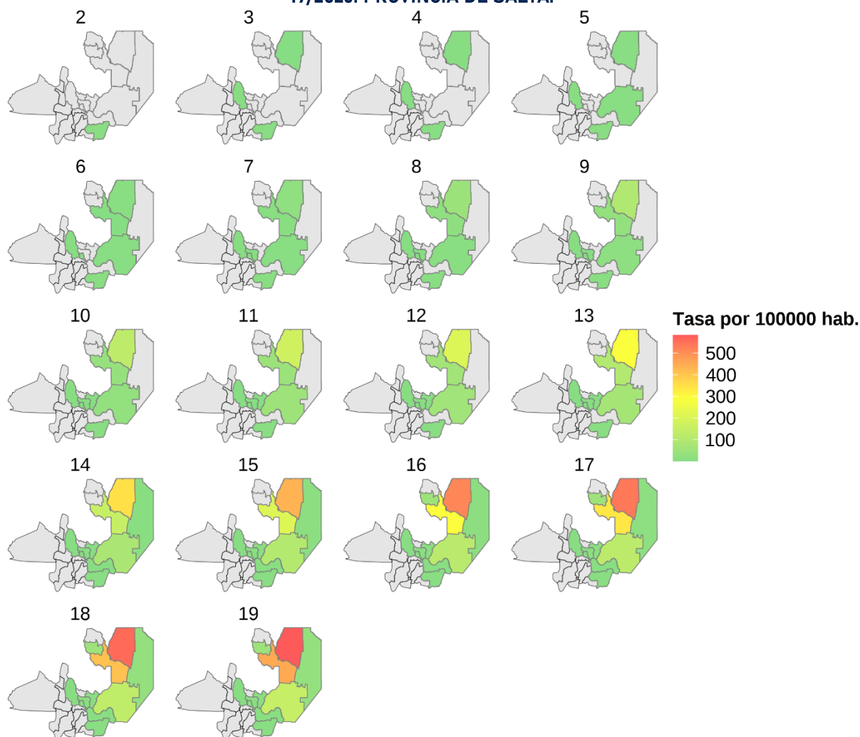
GRÁFICO 2.4. CHIKUNGUNYA: TASA DE INCIDENCIA ACUMULADA (POR 100.000 HAB.) POR DEPARTAMENTO, ACUMULADA HASTA CADA SEMANA EPIDEMIOLÓGICA. SE 2/2026 A SE 19/2026. PROVINCIA DE SALTA.
