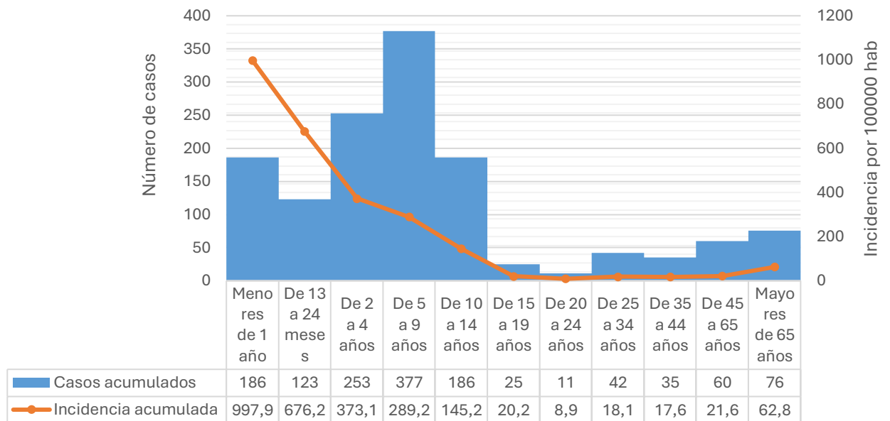
GRÁFICO N.º 3.20: DISTRIBUCIÓN DE CASOS Y TASA DE INCIDENCIA POR 100000 HAB. DE INTERNADOS POR IRA SEGÚN GRUPO DE EDAD. SE 1 HASTA SE 19. PROVINCIA DE SALTA. AÑO 2026
