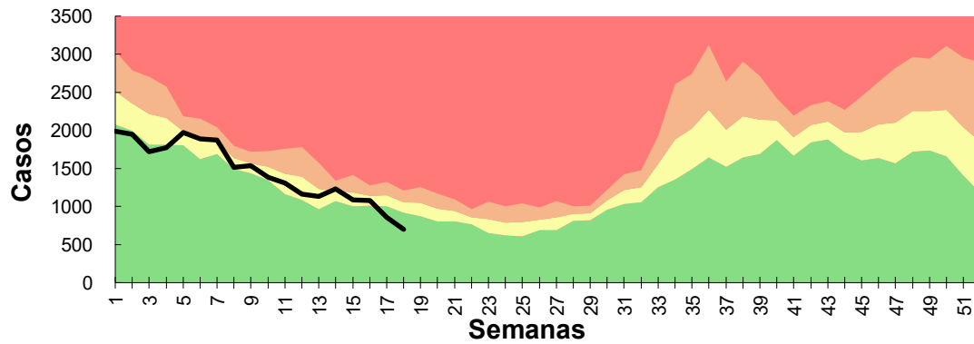
GRÁFICO 5.4. CORREDOR ENDÉMICO SEMANAL DE DIARREAS AÑOS: 2021 A 2025. SE 18 DE 2026. PROVINCIA DE SALTA. (n= 26.569)
