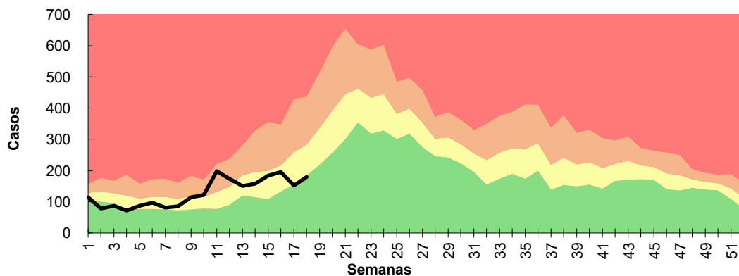
GRÁFICO 3.2. CORREDOR ENDÉMICO SEMANAL DE BRONQUIOLITIS EN MENORES DE 2 AÑOS AÑOS: 2019 A 2025. SE 18 DE 2026. PROVINCIA DE SALTA. (n=2.319)
