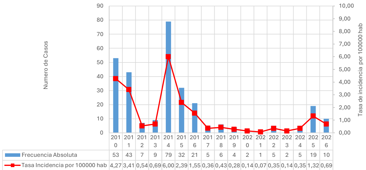
GRÁFICO 6.1. CASOS CONFIRMADOS DE HEPATITIS A Y TASA CADA 100MIL HAB. PERIODO 2010 HASTA SE 19/2026. PROVINCIA DE SALTA.
