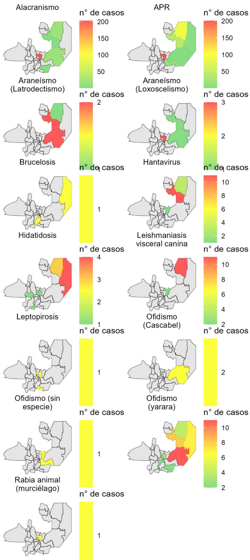
GRÁFICO 8.1. FRECUENCIA ACUMULADA DE CASOS CONFIRMADOS DE ENFERMEDADES ZONÓTICAS HUMANAS POR DEPARTAMENTO HASTA SE 19/2026. PROVINCIA DE SALTA.
