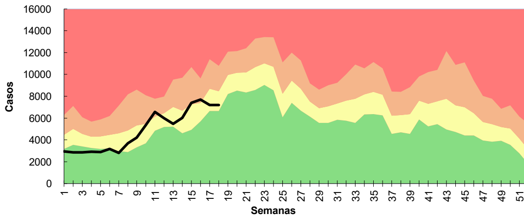
GRÁFICO 3.4. CORREDOR ENDÉMICO SEMANAL DE IRA AÑOS: 2019 A 2025. SE 18 DE 2026. PROVINCIA DE SALTA. (n=87.241)
