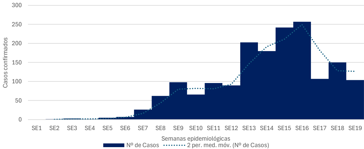
GRÁFICO 2.2. CHIKUNGUNYA: CASOS CONFIRMADOS POR SEMANA EPIDEMIOLÓGICA. (SE 1 HASTA SE 19). AÑO 2026. PROVINCIA DE SALTA (n=1698)
