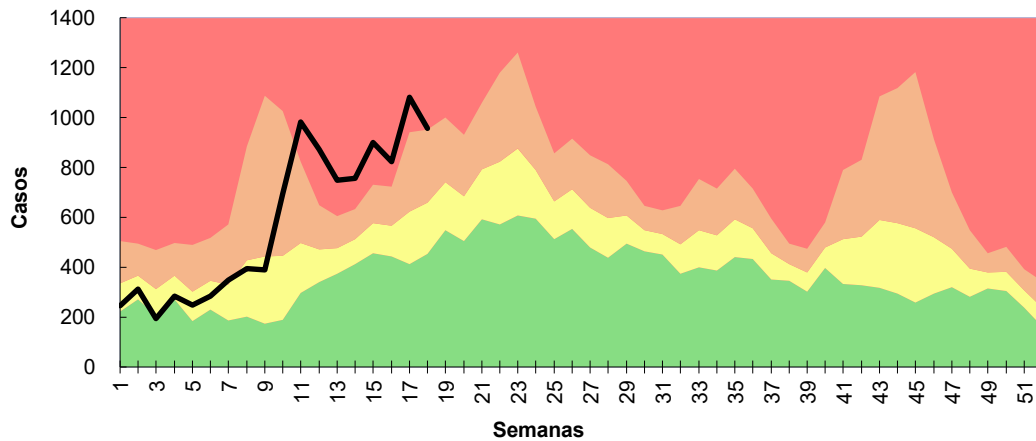
GRÁFICO 3.1. CORREDOR ENDÉMICO SEMANAL DE ENFERMEDAD TIPO INFLUENZA (ETI) – AÑOS: 2019 A 2025. SE 18 DE 2026. PROVINCIA DE SALTA. (n=10.508)
